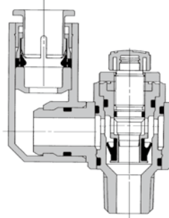
进气节流式 AS3311F-02
